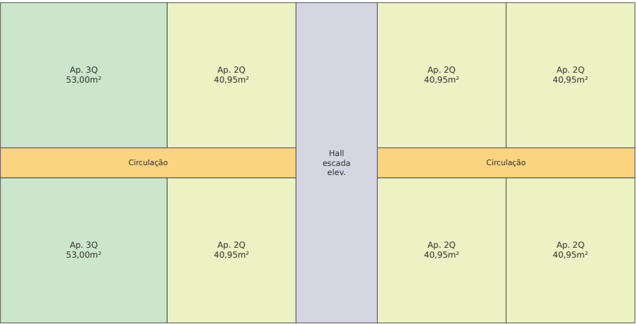
Pavimento Tipo 6 2Q + 2 3Q (8x)
